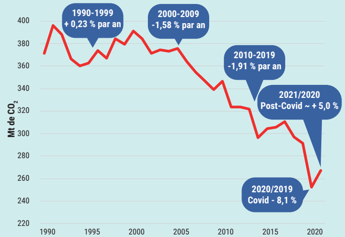
Émissions de CO 2 en France. Source : CITEPA (1990-2020) - Estimations diverses pour 2021.
